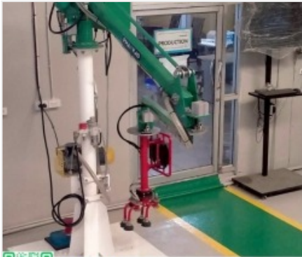
เครื่องช่วยยก Hybrid Manipulator รุ่น PKMS-75 PHAKKAD 02-079-1828
